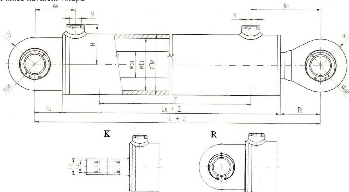
Rozměrová tabulka
